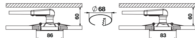
METALL - chrom inkl. 3W LED GU10 270lm 7208-038 · 3er-Set
