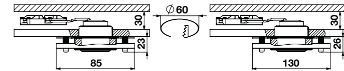
KUNSTSTOFF - matt-nickel / Acryl inkl. 5W LED-Modul 400lm 7216-012 · 1er
